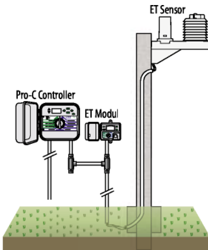
Der ET-Sensor kann bequem an Wand oder Pfosten bis zu einer Entfernung von 30 m installiert werden.
